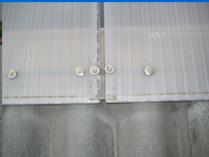
Montering af H-liste husk silikone i toppen
