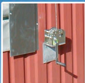
Foldegardiner betjent af manual reguleringshåndtag
