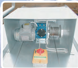
Foldegardin med RS850 gearmotor til automatisk regulering af gardiner. Tilkobles enten vejrcomputer SKY4 eller manuel reguleringsboks
